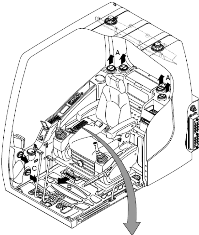
Панель переключателей
