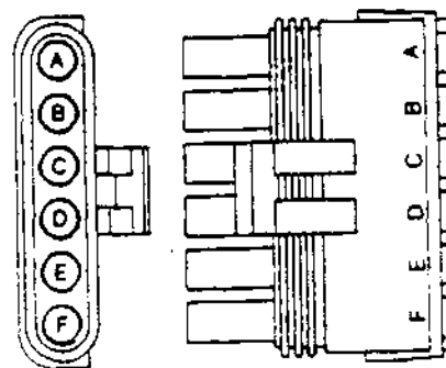
(Разъем X9)
