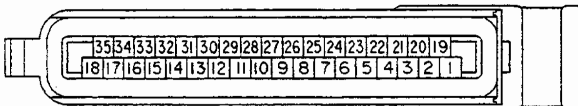
Разъем X1
